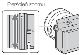
Pierścień zoomu Dźwignia zoomu (tylko w obiektywach z zoomem elektrycznym)
